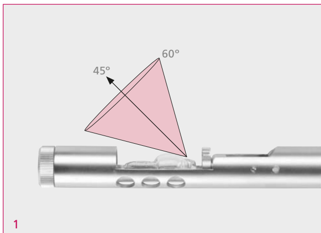
Abb. 1 Objektivkopf eines verlängerbaren Endoskopes mit Warmlicht Blickrichtung 45° – Blickfeld 60°
