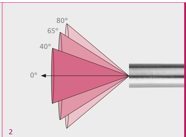
Abb. 2 verschiedene Blickfelder eines Kaltlicht-Endoskopes mit einer Blickrichtung von 0°
