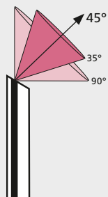
Darstellung der unterschiedlichen Blickrichtungen und -winkel von starren Endoskopen Representation of the different viewing directions and angles of rigid borescopes
