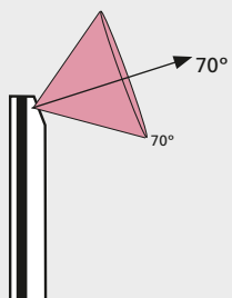
Darstellung der unterschiedlichen Blickrichtungen und -winkel von starren Endoskopen Representation of the different viewing directions and angles of rigid borescopes
