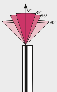
Darstellung der unterschiedlichen Blickrichtungen und -winkel von starren Endoskopen Representation of the different viewing directions and angles of rigid borescopes
